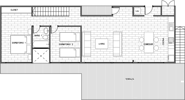
PLANTA ARQUITECTURA 1 PISO
