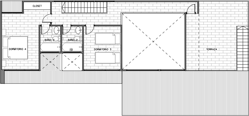
PLANTA ARQUITECTURA 2 PISO
