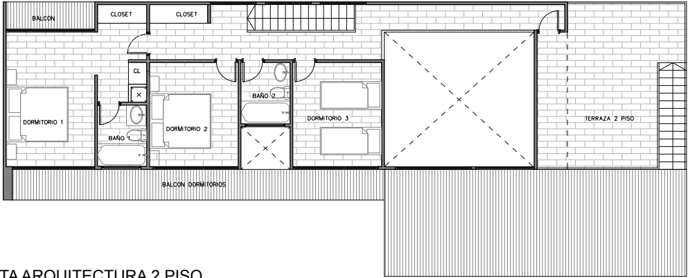
PLANTA ARQUITECTURA 2 PISO
