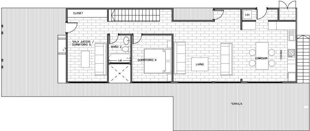
PLANTA ARQUITECTURA 1 PISO
