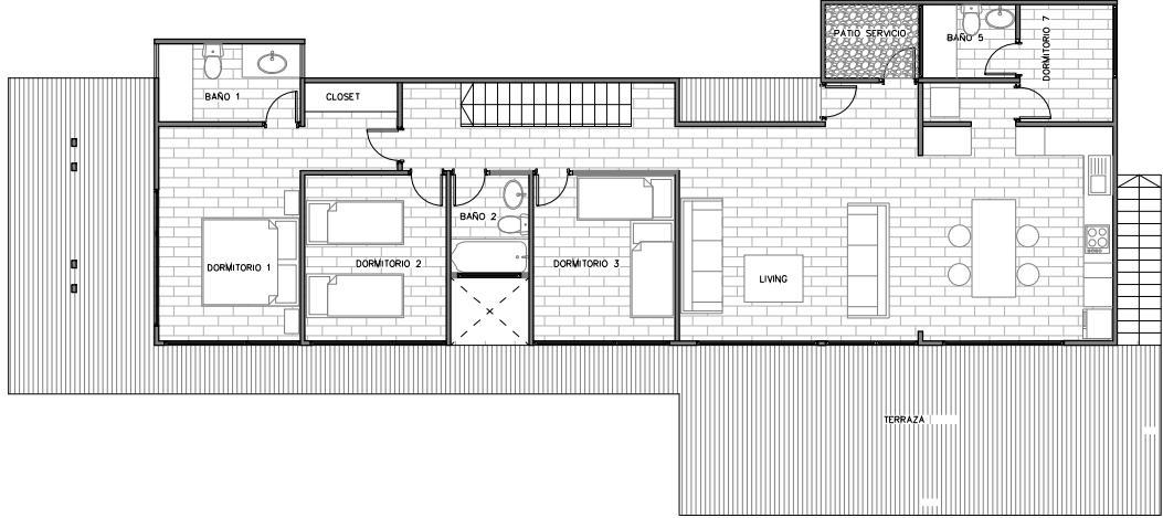
PLANTA ARQUITECTURA 1 PISO
